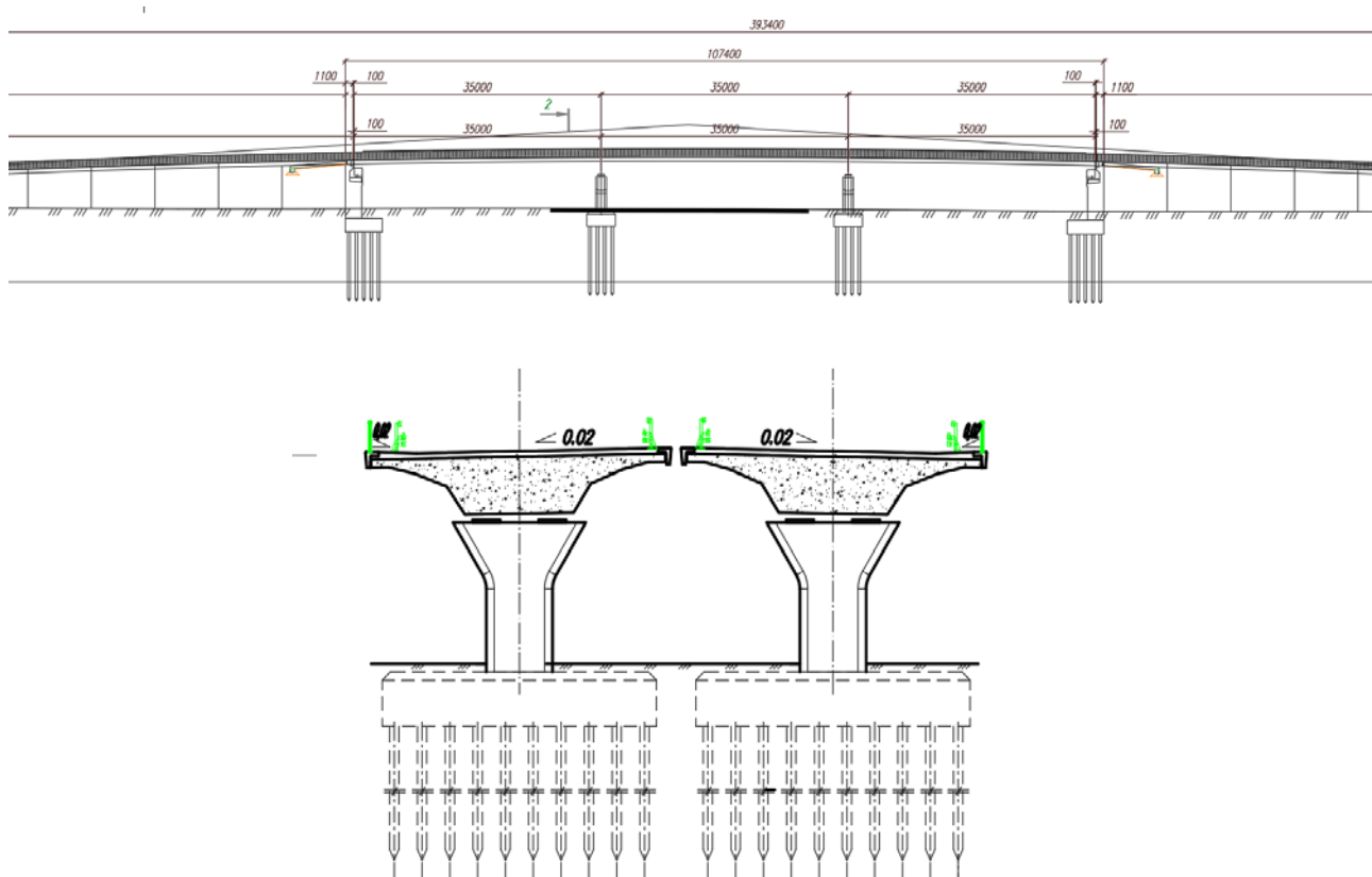
Рисунок 24 – Типовое решение транспортного сооружения в продольном и поперечном профилях
