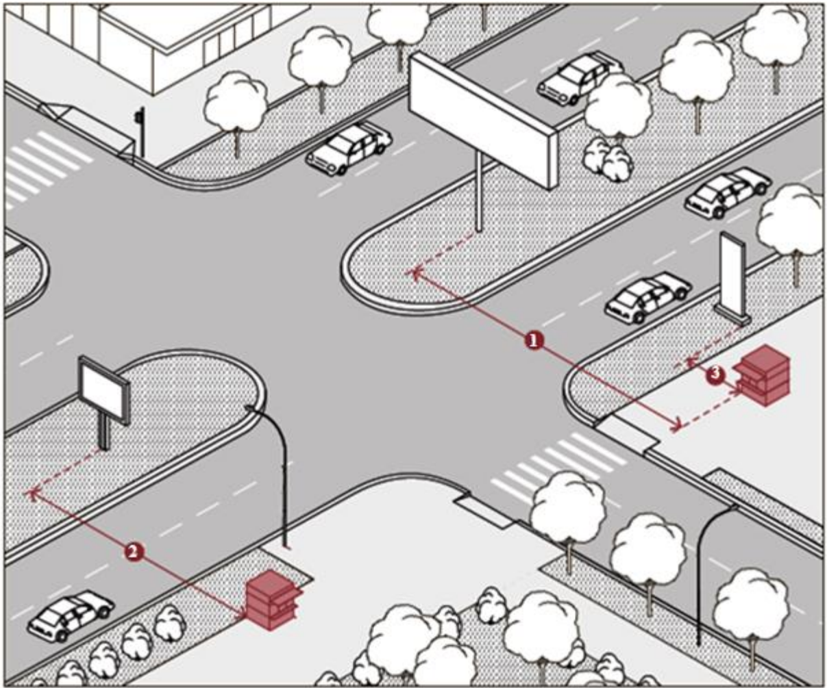
Рисунок 8. Размещение НТО относительно рекламных конструкций
