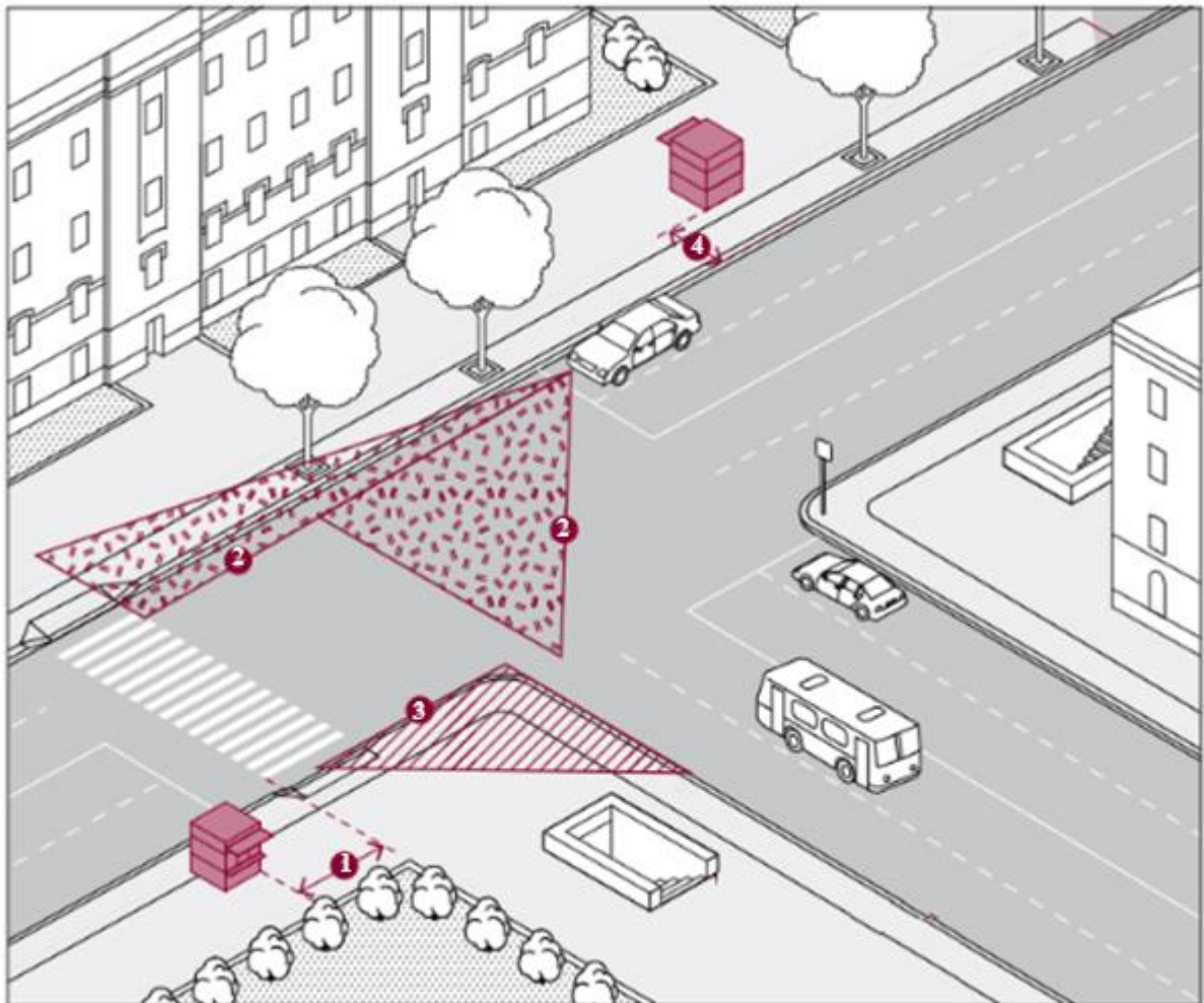
Рисунок 6. Размещение НТО относительно элементов улично-дорожной сети
